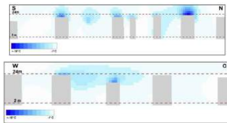
Bsp.: Simulierte Lufttemperaturen über intensiv begrünten Dächern Grafik bereitgestellt durch: GEO-NET Umweltconsulting GmbH
