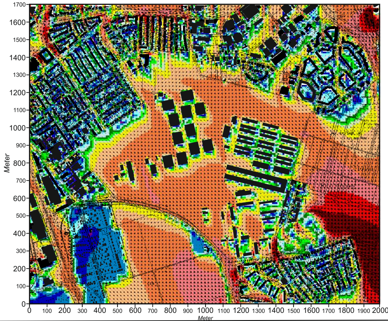
Abb. 15.1 Ist-Zustand - Belüftungsverhältnisse 2 m ü.G., Windanströmung aus Nordnordwesten mit 2.0 m/s in einer Höhe von 10 m ü.G.
