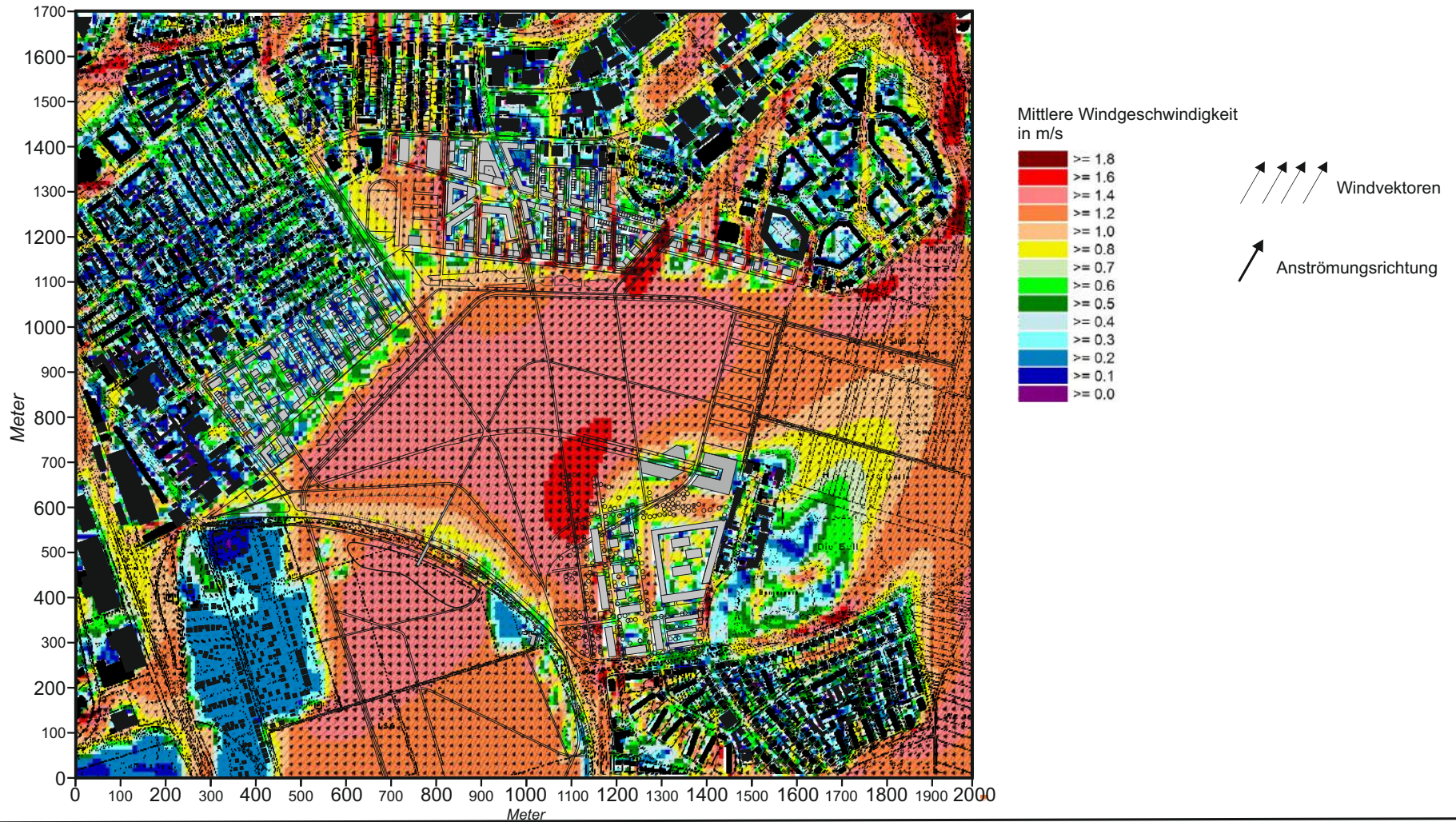
Abb. 14.2 Plan-Zustand - Belüftungsverhältnisse 2 m ü.G., Windanströmung aus Südsüdwesten mit 2.0 m/s in einer Höhe von 10 m ü.G.
