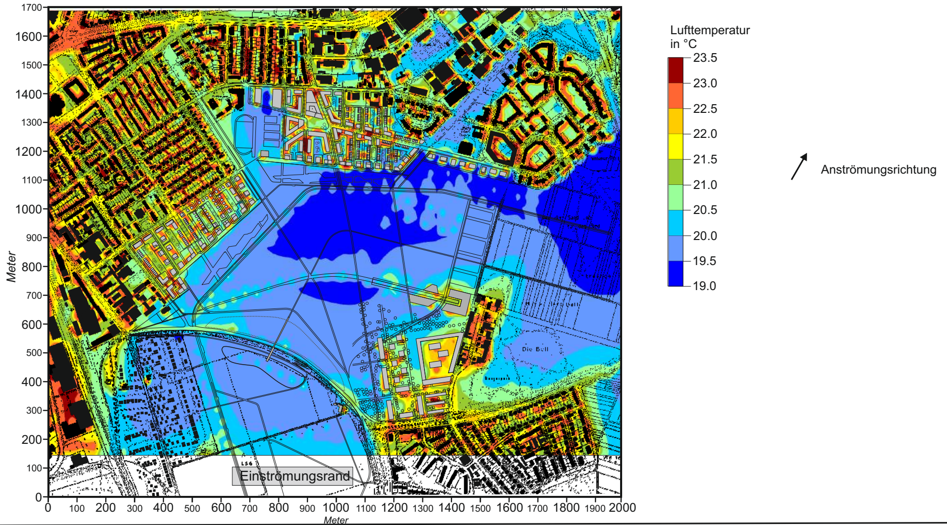
Abb. 18.2 Plan-Zustand - Lufttemperaturverteilung 2 m ü.G. in einer warmen Sommernacht (02:00 Uhr), Windanströmung aus Südsüdwesten mit 1.0 m/s in einer Höhe von 10 m ü.G.
