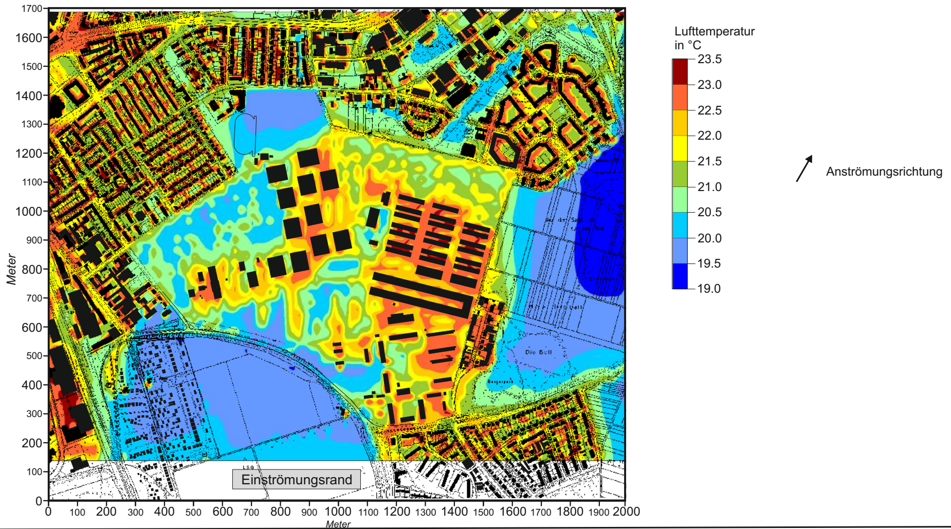
Abb. 18.1 Ist-Zustand - Lufttemperaturverteilung 2 m ü.G. in einer warmen Sommernacht (02:00 Uhr), Windanströmung aus Südsüdwesten mit 1.0 m/s in einer Höhe von 10 m ü.G.
