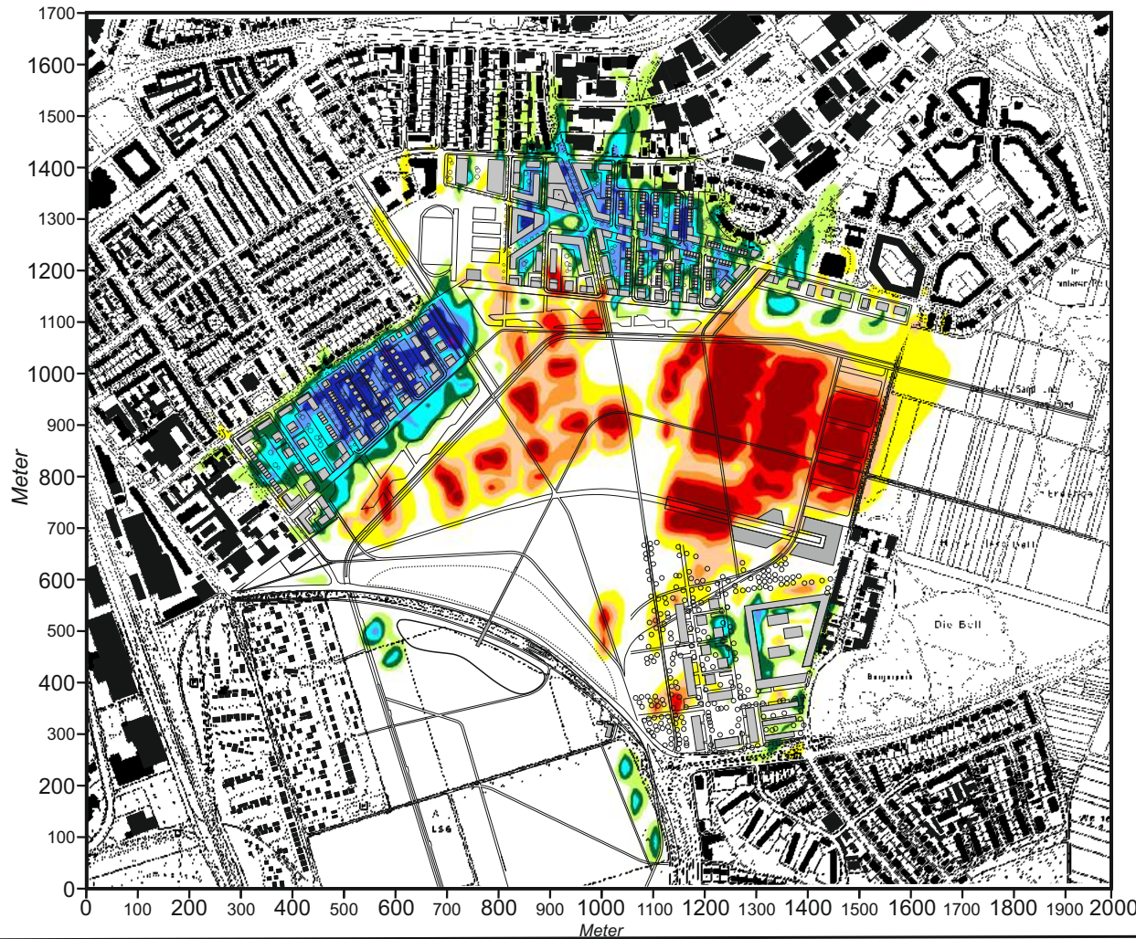
Abb. 14.3 Veränderung der Belüftungsverhältnisse 2 m ü.G. durch den Plan-Zustand gegenüber dem Ist-Zustand, Windanströmung aus Südsüdwesten mit 2.0 m/s in einer Höhe von 10 m ü.G.
