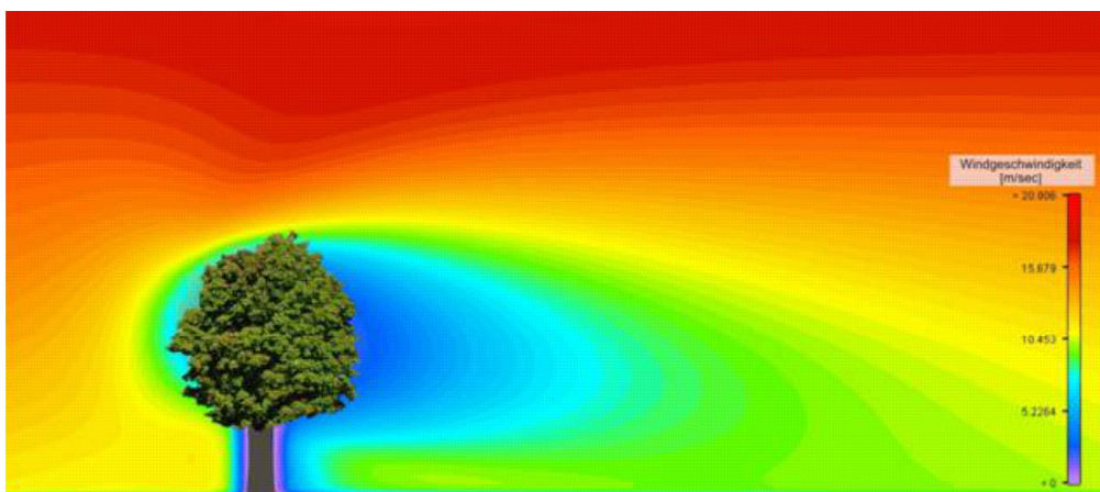
Grafik 1: Hinderniswirkung eines Einzelbaums – Ergebnis numerischer Modellrechnungen. © Institut für Hydromechanik – KIT Karlsruhe, Prof. Dr. Bodo Ruck (Leiter der Arbeitsgruppe Gebäude- und Umweltaerodynamik).
