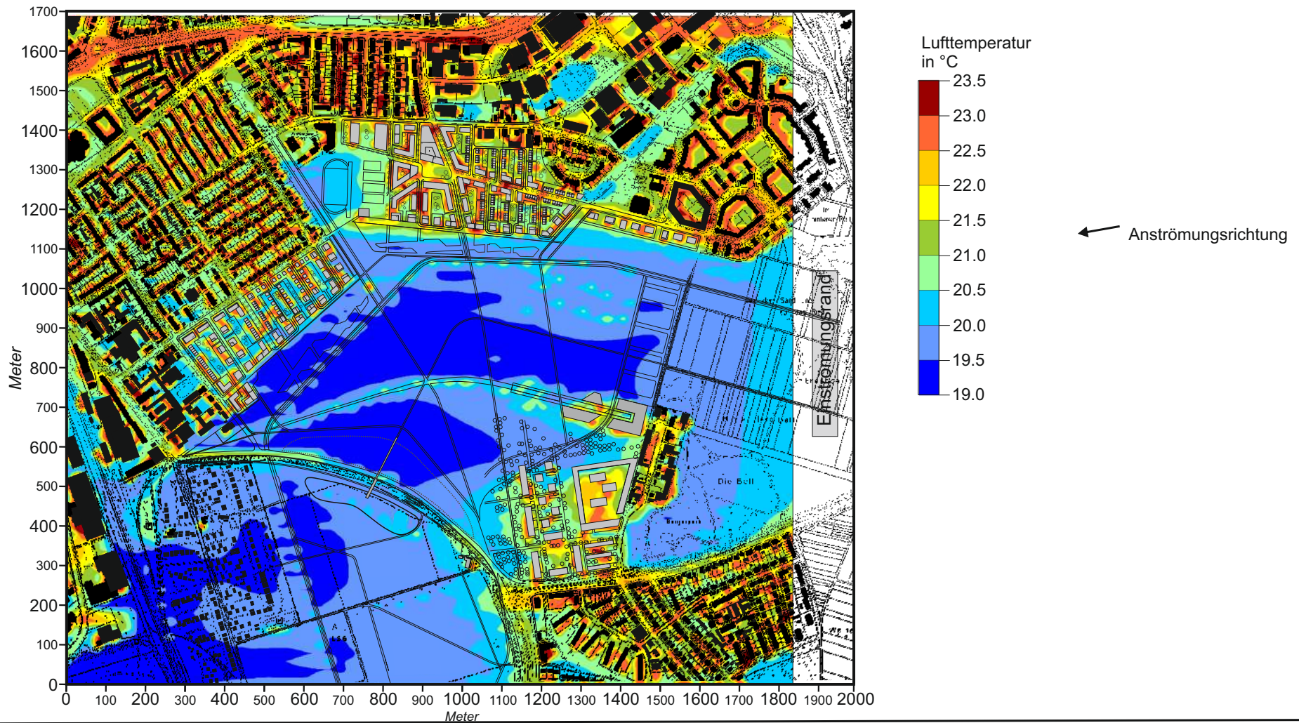
Abb. 19.2 Plan-Zustand - Lufttemperaturverteilung 2 m ü.G. in einer warmen Sommernacht (02:00 Uhr), Windanströmung aus Osten mit 1.0 m/s in einer Höhe von 10 m ü.G.
