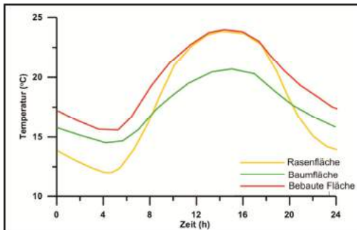
Bsp.: Temperaturverlauf im Bereich einer Baumfläche im Vergleich zu unbeschatteten Flächen.
