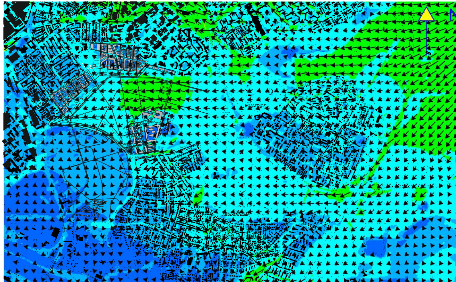
Abb. 12.1 Plan-Zustand / Kaltluftbewegungen (02:00 Uhr) - Kaltluft-Fließgeschwindigkeit und Strömungsrichtung (Schichtmittel 0 - 4 m ü.G.) in einer windschwachen Strahlungsnacht. Ergebnisse mesoskaliger Modellrechnungen
