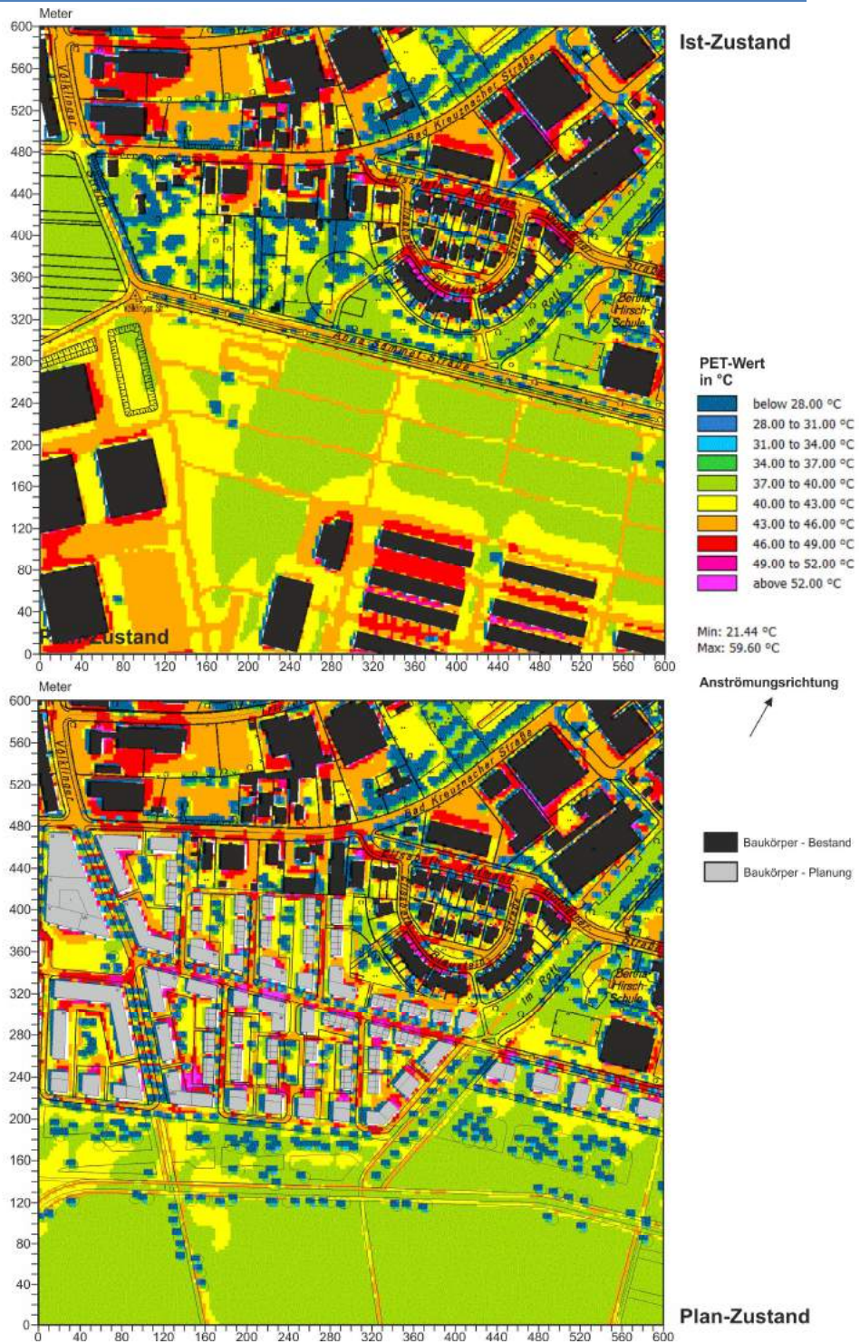
Grafik 3: Vergleich zwischen Ist- und Plan-Zustand. PET-Wert an einem warmen Sommertag gegen 17:00 Uhr (Lufttemperatur ~ 27°C)
