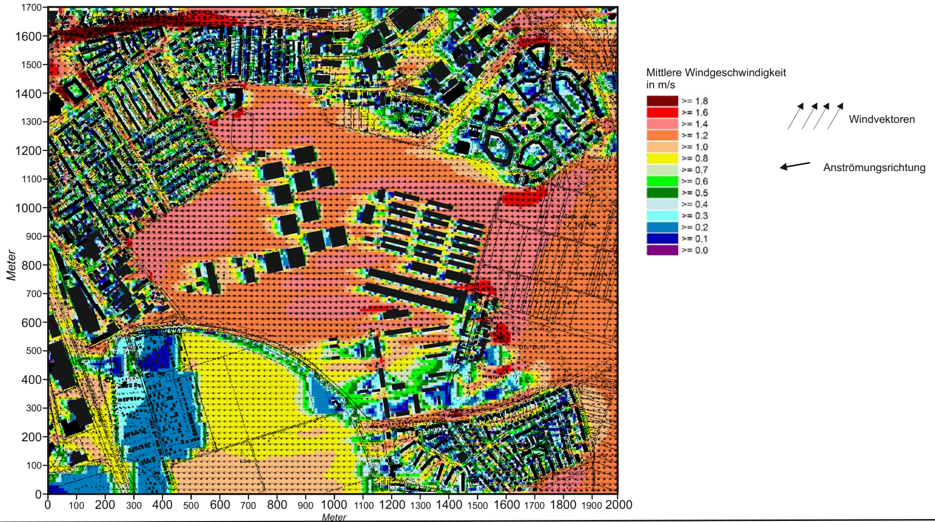
Abb. 16.1 Ist-Zustand - Belüftungsverhältnisse 2 m ü.G., Windanströmung aus Osten mit 2.0 m/s in einer Höhe von 10 m ü.G.
