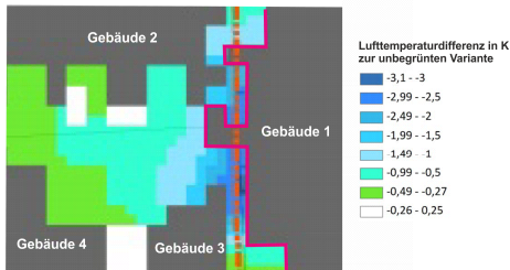
— Fassadenbegrünung Bsp.: Simulierte Lufttemperaturen in einem Innenhof Grafik aus: GEO-NET Umweltconsulting GmbH, ÖKOPLANA 2017
