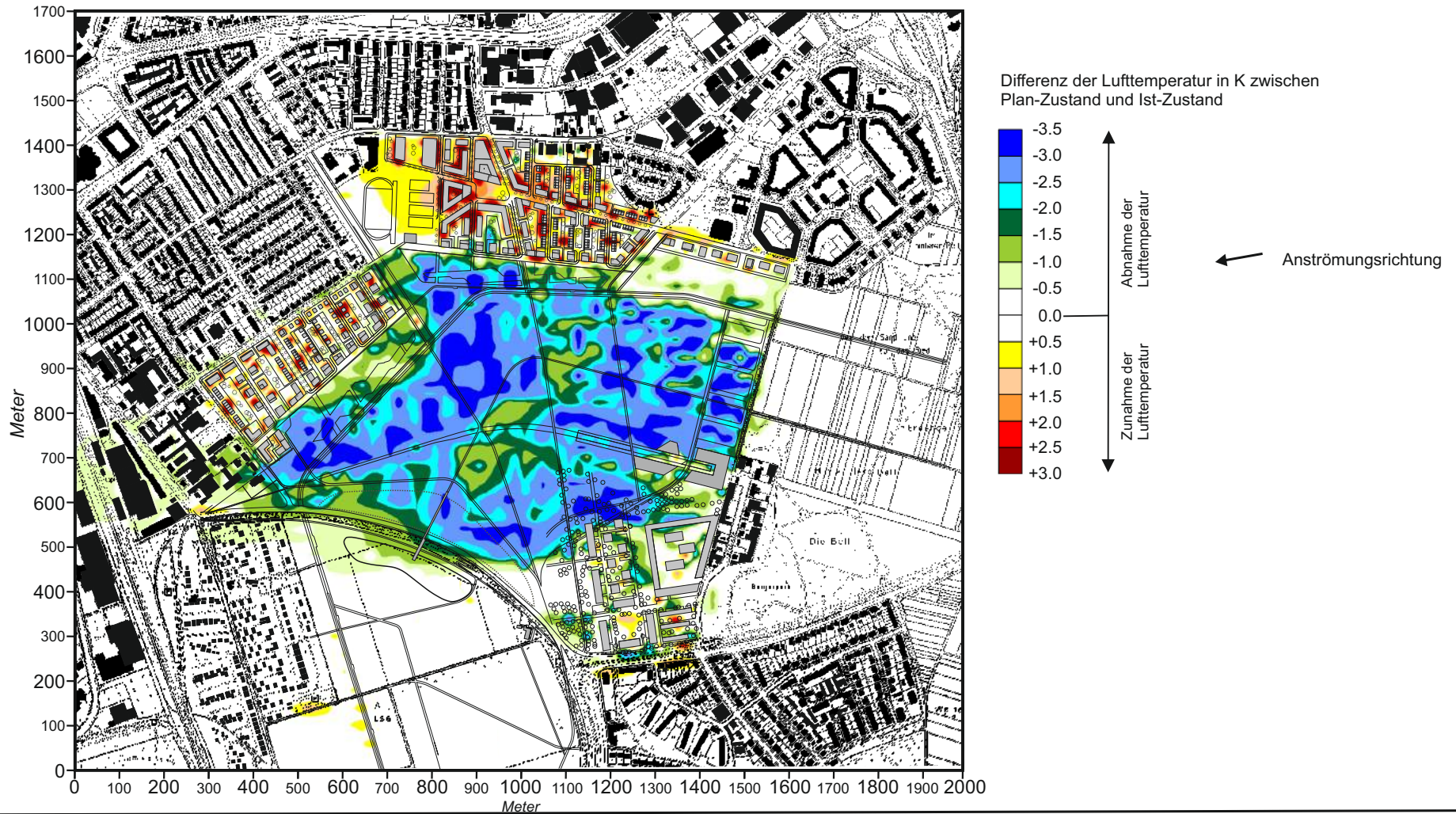
Abb. 19.3 Veränderung der Lufttemperaturverteilung 2 m ü.G. durch den Plan-Zustand gegenüber dem Ist-Zustand. Windanströmung aus Osten mit 1.0 m/s in einer Höhe von 10 m ü.G.
