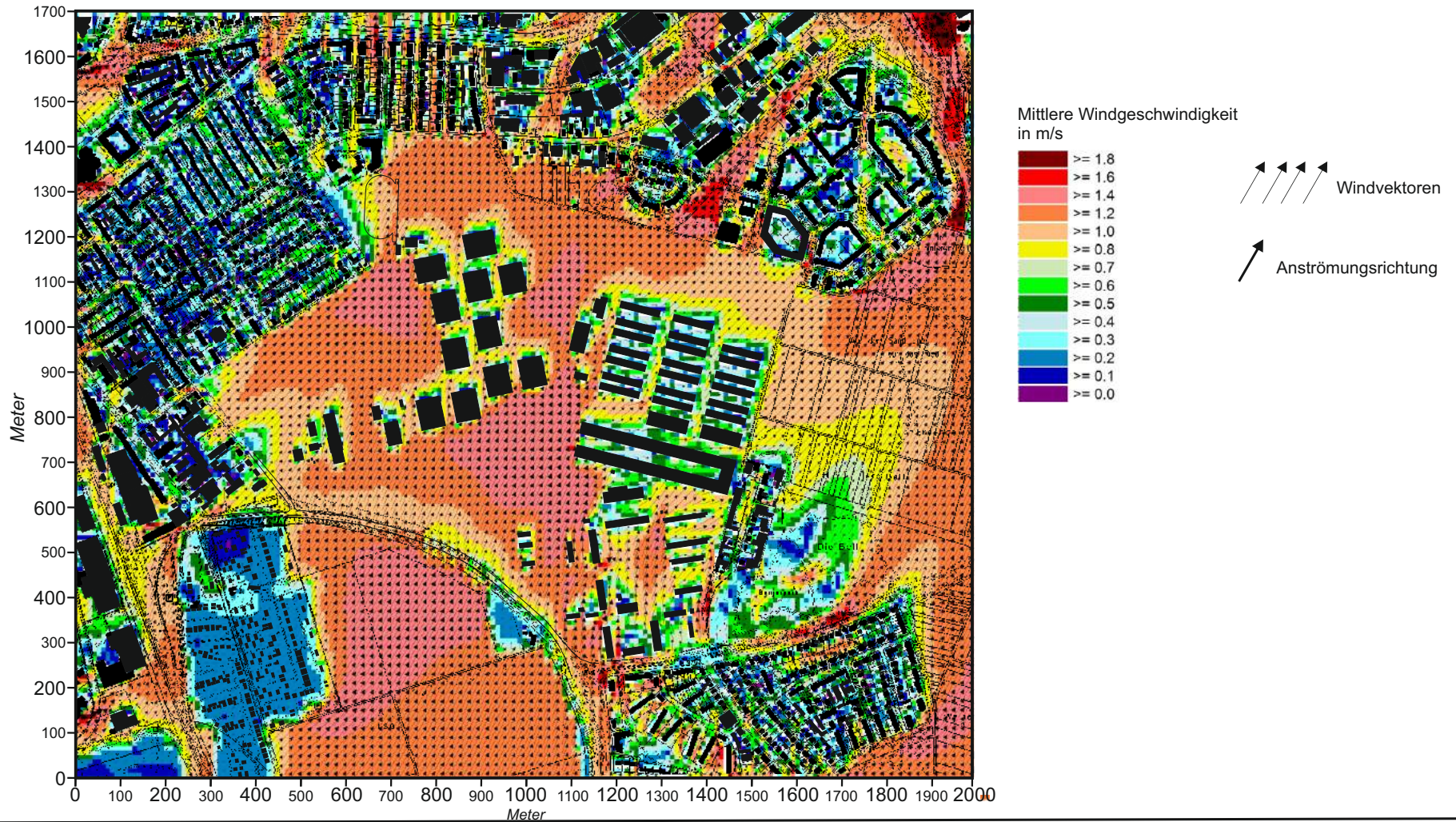
Abb. 14.1 Ist-Zustand - Belüftungsverhältnisse 2 m ü.G., Windanströmung aus Südsüdwesten mit 2.0 m/s in einer Höhe von 10 m ü.G.
