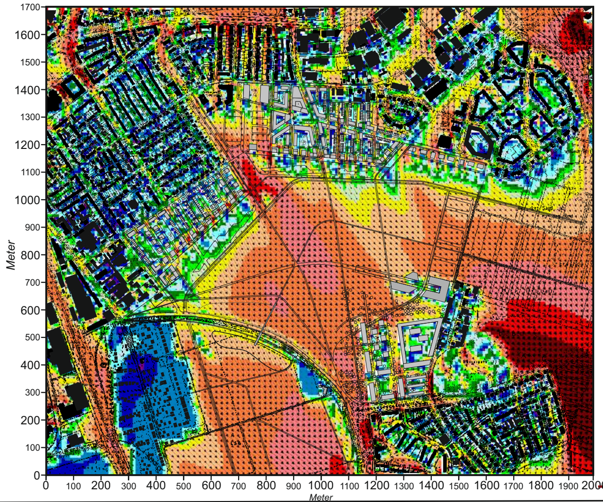
Abb. 15.2 Plan-Zustand - Belüftungsverhältnisse 2 m ü.G., Windanströmung aus Nordnordwesten mit 2.0 m/s in einer Höhe von 10 m ü.G.
