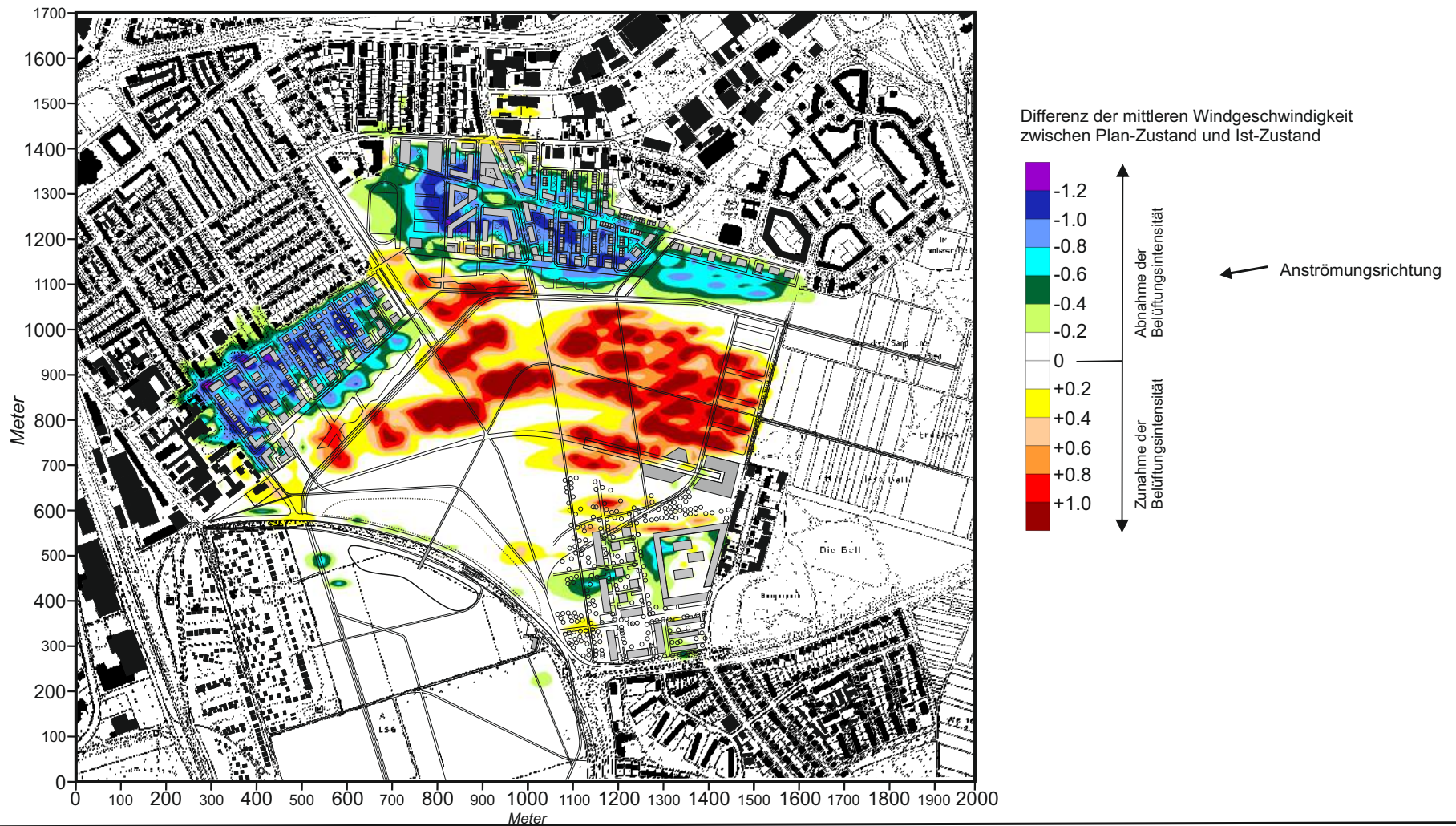
Abb. 16.3 Veränderung der Belüftungsverhältnisse 2 m ü.G. durch den Plan-Zustand gegenüber dem Ist-Zustand, Windanströmung aus Osten mit 2.0 m/s in einer Höhe von 10 m ü.G.
