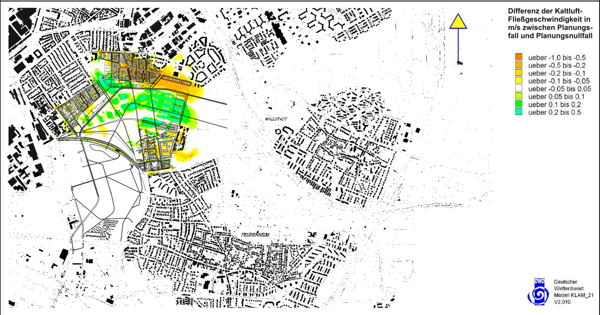
Abb. 13.1 Plan-Zustand / Kaltluftbewegungen (02:00 Uhr) - Differenz der Kaltluft-Fließgeschwindigkeit (Schichtmittel 0 - 4 m ü.G.) zum Ist-Zustand in einer windschwachen Strahlungsnacht. Ergebnisse mesoskaliger Modellrechnungen
