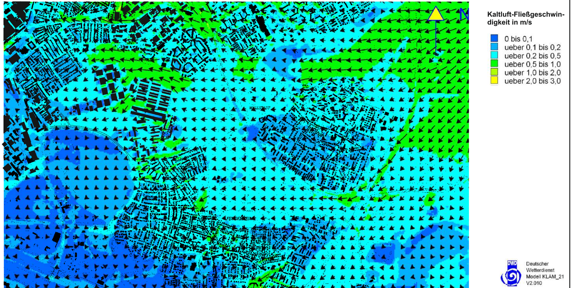
Abb. 11.1 Ist-Zustandl / Kaltluftbewegungen (02:00 Uhr) - Kaltluft-Fließgeschwindigkeit und Strömungsrichtung (Schichtmittel 0 - 4 m ü.G.) in einer windschwachen Strahlungsnacht. Ergebnisse mesoskaliger Modellrechnungen
