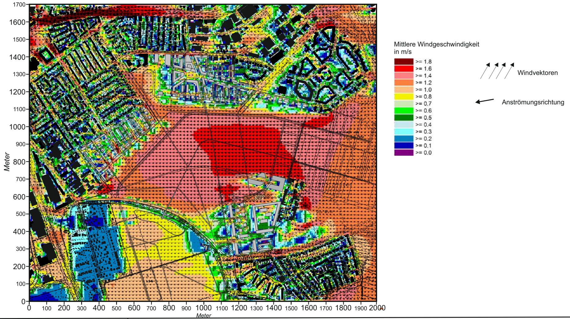
Abb. 16.2 Plan-Zustand - Belüftungsverhältnisse 2 m ü.G., Windanströmung aus Osten mit 2.0 m/s in einer Höhe von 10 m ü.G.
