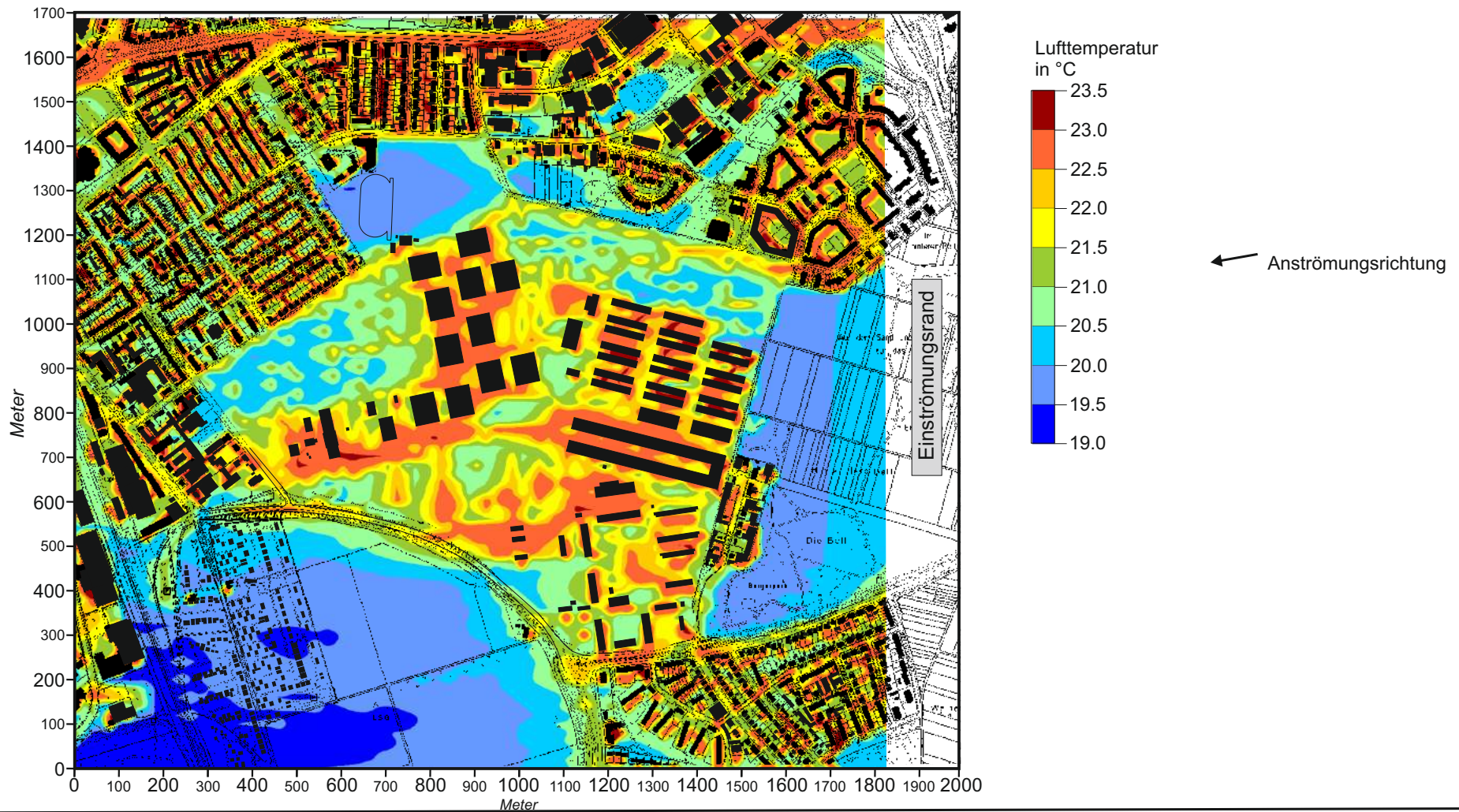
Abb. 19.1 Ist-Zustand - Lufttemperaturverteilung 2 m ü.G. in einer warmen Sommernacht (02:00 Uhr), Windanströmung aus Osten mit 1.0 m/s in einer Höhe von 10 m ü.G.
