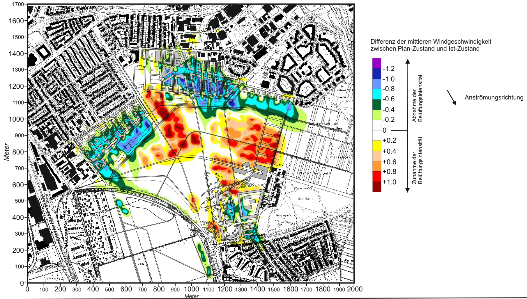
Abb. 15.3 Veränderung der Belüftungsverhältnisse 2 m ü.G. durch den Plan-Zustand gegenüber dem Ist-Zustand, Windanströmung aus Nordnordwesten mit 2.0 m/s in einer Höhe von 10 m ü.G.
