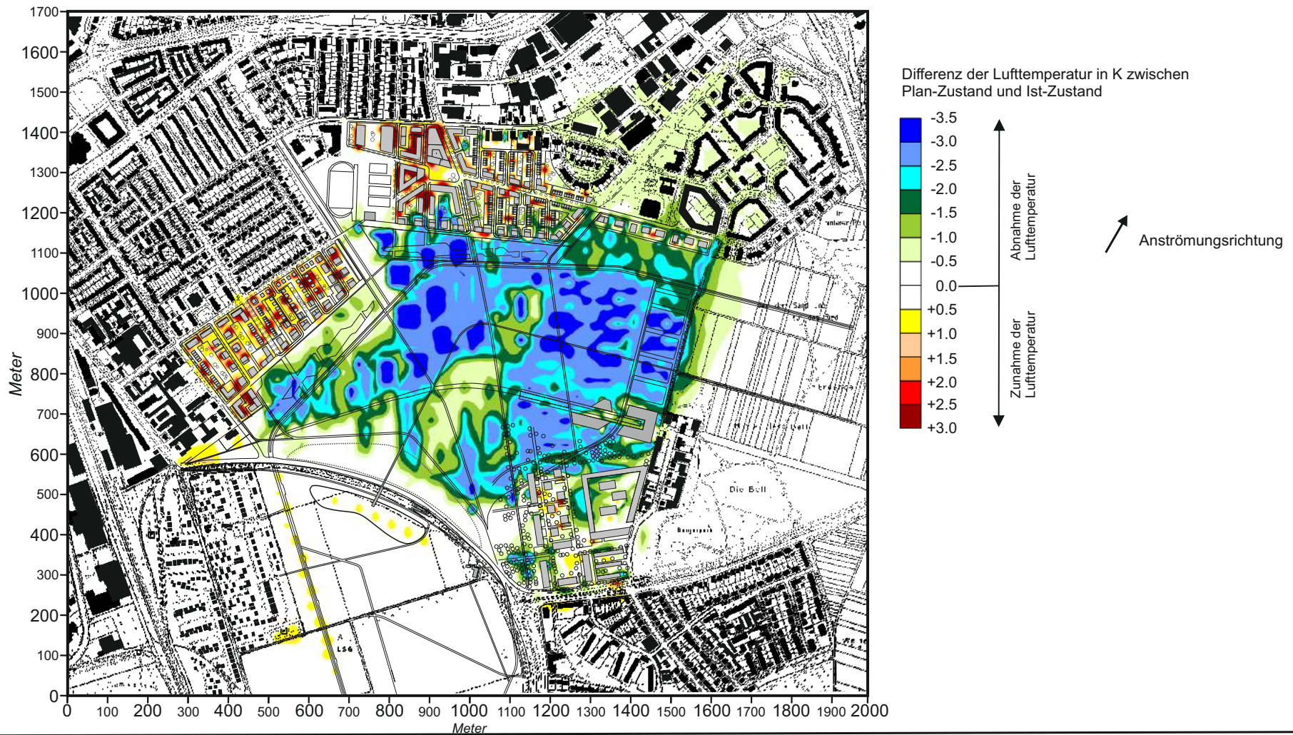
Abb. 18.3 Veränderung der Lufttemperaturverteilung 2 m ü.G. durch den Plan-Zustand gegenüber dem Ist-Zustand. Windanströmung aus Südsüdwesten mit 1.0 m/s in einer Höhe von 10 m ü.G.
